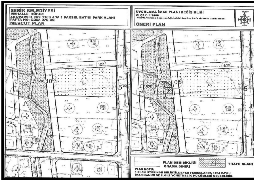
Şekil 43 : Kökeç Mahallesi 1163 Ada 1 Parselin Batısında Bulunan Park Alanına Trafo Konulması 1/1000 Ölçekli Uygulama İmar Planı Değişikliği
